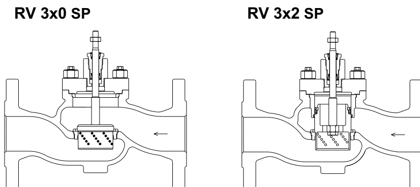
Obr.1: Směr proudění dvoucestnou armaturou s válcovou nebo tvarovanou kuželkou RV 3xx xxx xxxx Lx xx/xxx-xxx SP (Char. L; R; P; S; U)
