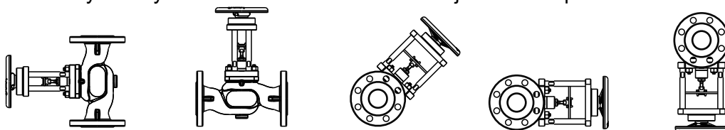
Obr.5: Montážní polohy ventilů s ručním kolem
