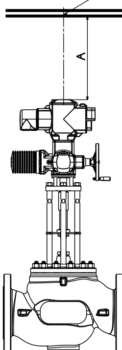
Obr.6: Manipulační prostor nad ventilem
