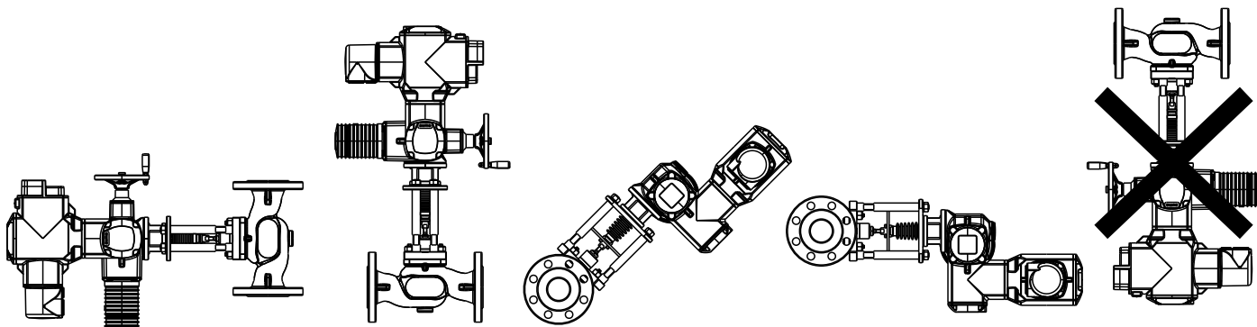
Obr.3: Montážní polohy ventilů s elektrickými pohony
