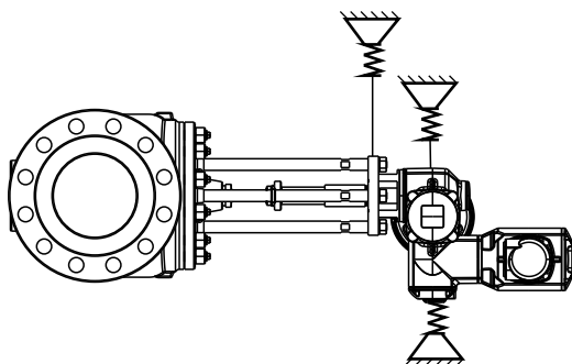
Obr.7: Doporučená místa vhodná pro ukotvení
