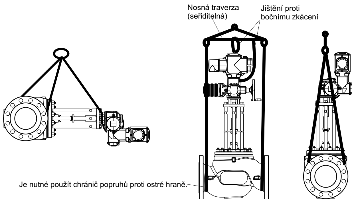
Obr.8: Příklad použití vázacích prostředků při manipulaci
