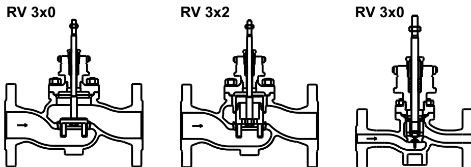
Рис. 1: Направление потока через двухходовую арматуру с цилиндрическим или форматированным конусом RV 2xx xxx xxxx Lx xx/xxx-xxx (Харак. L; R; P; S; U)
