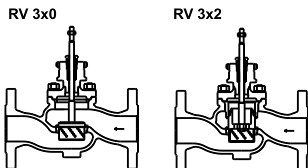
Рис. 2: Направление потока через двухходовую арматуру с перфорированным конусом RV 3xx xxx xxxx Dx xx/xxx-xxx (Харак. D; Z; Q)
