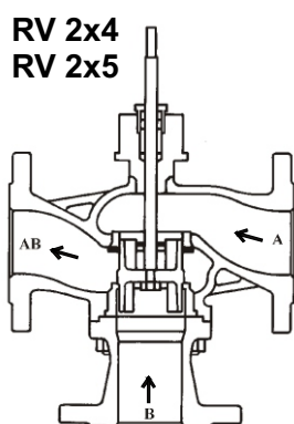
Рис. 3: Направление потока через трехпутевую арматуру со смесительной функцией
