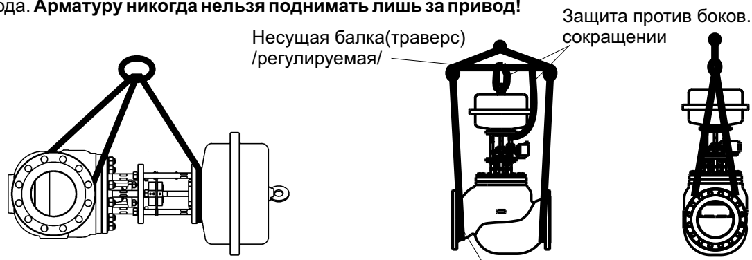
Рис. 10: Пример использования такелажных средств при манипулировании с устройством
