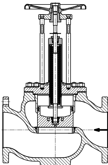
Obr.2: Směr proudění armaturou s tlakově odlehčenou kuželkou
